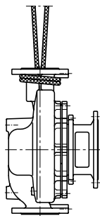
Obr. 2: Přeprava čerpadla
