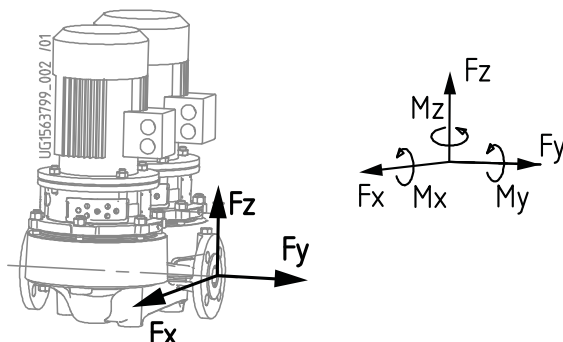
Obr. 6: Síly a momenty u hrdel čerpadla
