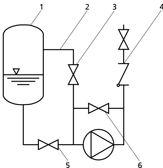
Obr. 7: Vyrovnání vakua
