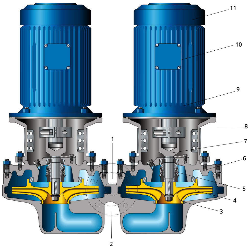
Obr. 4: Průřez
