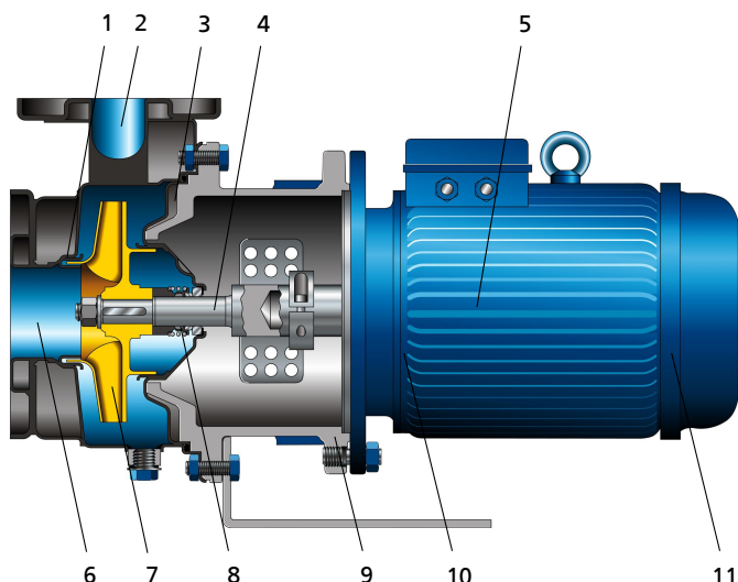
Obr. 7: Průřez
