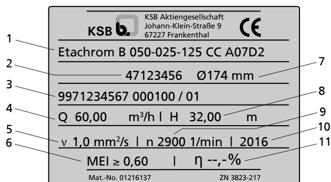
Obr. 6: Typový štítek Etachrom BC (příklad)
