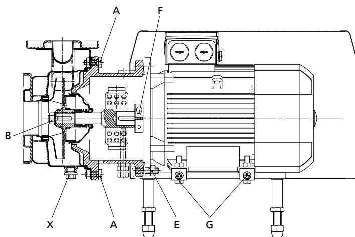
Obr. 20: Místa pro utahení šroubů pro Etachrom B 050-025-125.1, 050-025-125, 050-025-160, 050-025-200, 050-032-125.1, 050-032-125, 050-032-160, 050-032-200, 065-040-125, 065-040-160, 065-040-200, 065-050-125, 065-050-160
