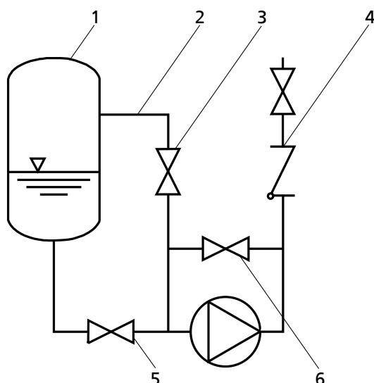
Obr. 10: Vyrovnání vakua
