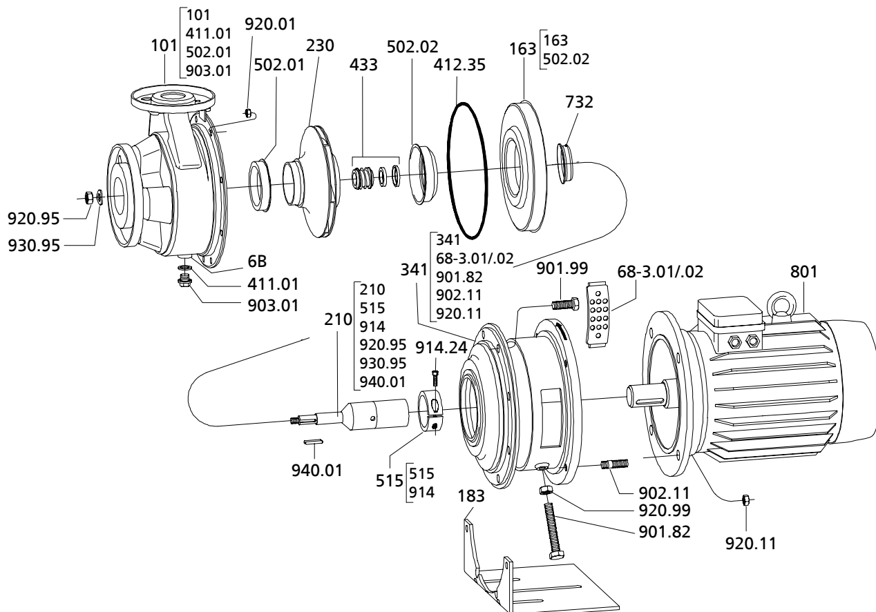
Obr. 23: Rozložené zobrazení provedení s hřídelovou jednotkou 25.1
