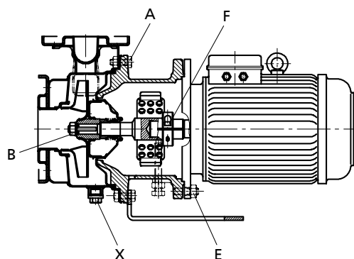
Obr. 19: Místa pro utahení šroubů pro Etachrom B 050-025-125.1, 050-025-125, 050-025-160, 050-025-200, 050-032-125.1, 050-032-125, 050-032-160, 050-032-200, 065-040-125, 065-040-160, 065-040-200, 065-050-125, 065-050-160
