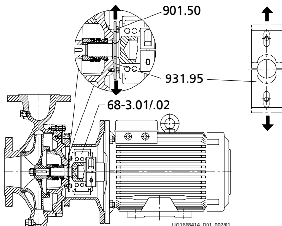
Obr. 12: Odstraňte pojistný plech
