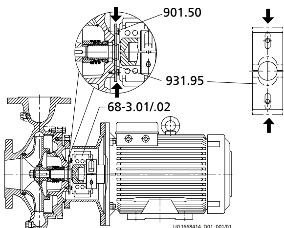
Obr. 14: Montáž pojistného plechu
