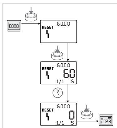
Fig. 56: Квітування помилок типу А або D
