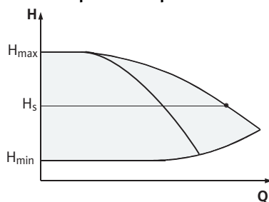
Fig. 19: Регулювання \Delta p -с (режим паралельної роботи)
