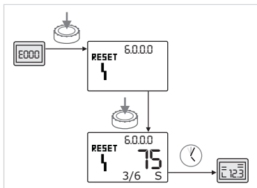
Fig. 58: Квитування помилок типу В (X < Y)
