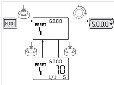
Fig. 53: Навігація по випадках помилок
