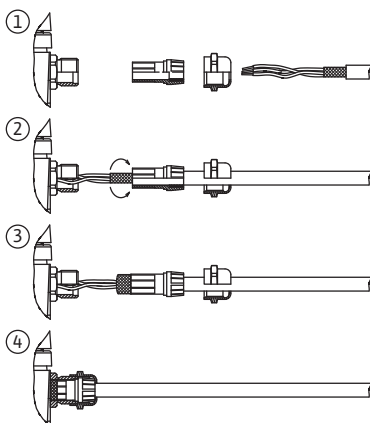
Fig. 28: Екранування кабелю
