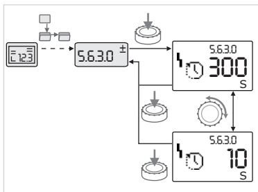
Fig. 41: Налаштування з поверненням до елемента меню «Вибір/налаштування»
