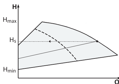
Fig. 20: Регулювання \Delta p -v (режим паралельної роботи)
