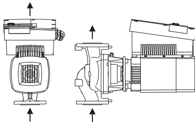
Fig. 22: Розташування компонентів у стані постачання
