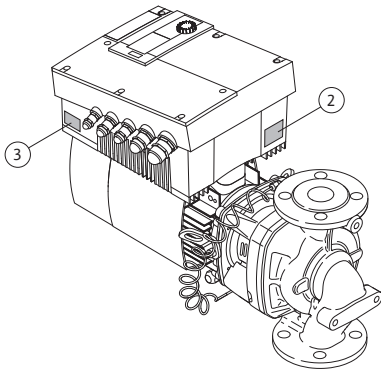
Fig. 12: Розміщення заводських табличок: Заводська табличка приводу, заводська табличка електронного модуля
