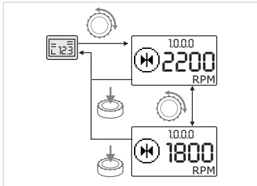
Fig. 36: Уведення заданого значення
