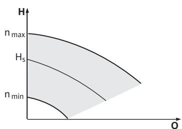
Fig. 47: Режим керування
