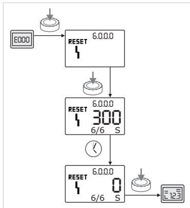
Fig. 59: Квитування помилок типу B ( X = Y )
