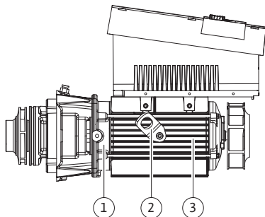
Fig. 13: Модуль
