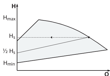
Fig. 16: Регулювання Др-в
