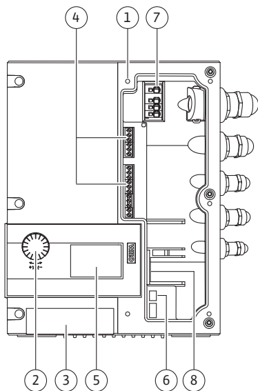
Fig. 14: Електронний модуль
