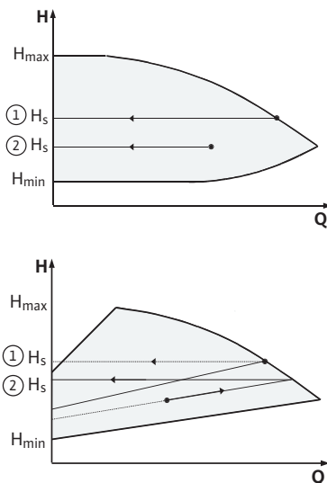
Fig. 46: Регулювання Др-с/Др-в
