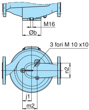
Фланцы PN 10, EN 1092-2
