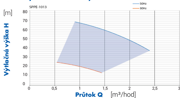
Hydraulická křivka výkonu
