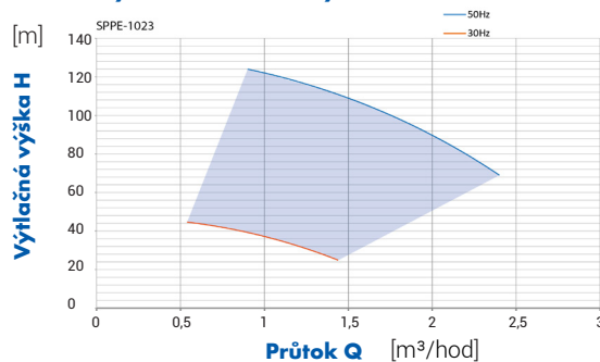
Hydraulická křivka výkonu
