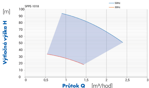
Hydraulická křivka výkonu
