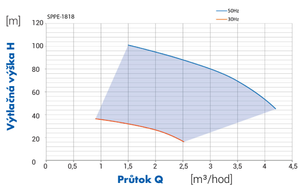
Hydraulická křivka výkonu
